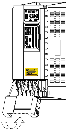
Рис. 3-7. Установка крышки
