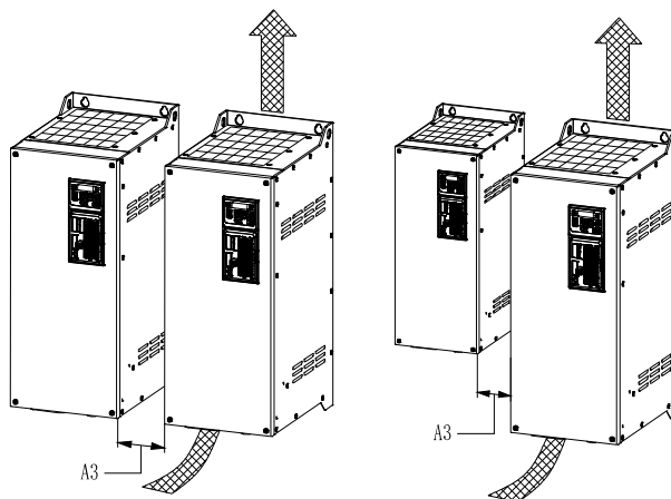
Рис. 3-3. Минимальные монтажные зазоры для приводов GK900-4T0.75LB – GK900-4T500L
