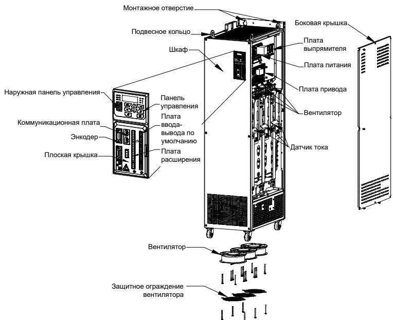
Рис. 2-3. Чертеж деталей
