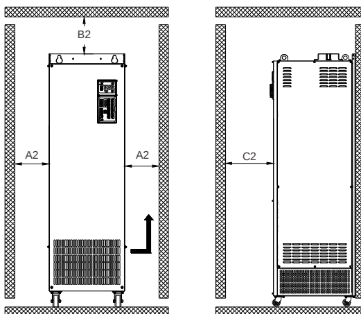
Рис. 3-2. Монтажные зазоры для приводов GK900-4T250G – GK900-4T450G
