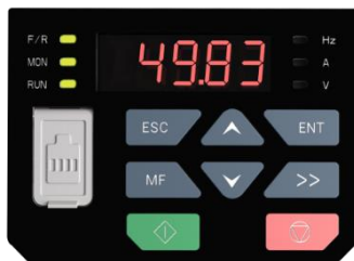
Рис. 4-6. Режим установки значения параметра (для b0-02 установлено 49,83 Гц)
