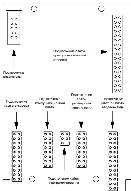
Рис. 3-23. Схема платы управления
