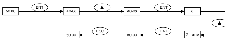
Рис. 4-13. Блок-схема инициализации параметров пользователя
