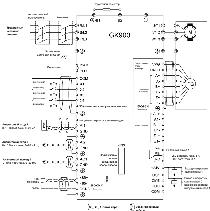
Рис. 3-24. Схема подключения
