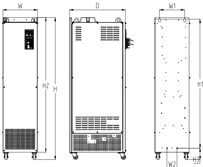
Рис. 2-4. Наружные размеры
